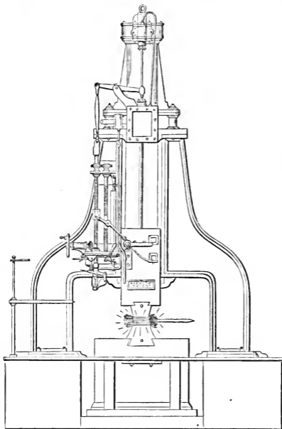
Fig. 4.—Steam-hammer.
